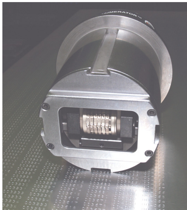
3-1/2" D-työkalupidin, jossa integroitu pituudensäätö ja neljä ulkopuolista kiilauraa joustavuuden maksimoimiseksi.
